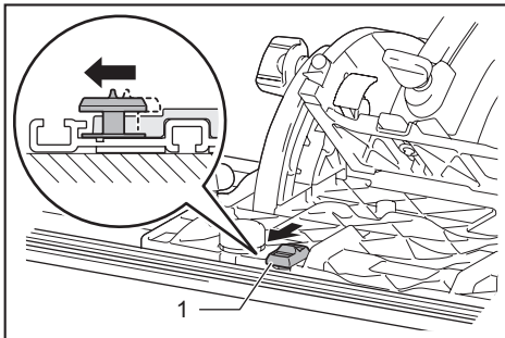
► 1. Palanca deslizante
